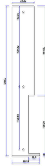
KESİM ŞABLONU CUTTING TEMPLATE
