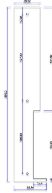
KESİM ŞABLONU CUTTING TEMPLATE
